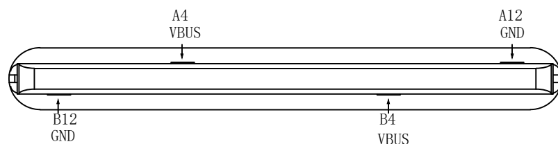
接点定义放大图(2P)
