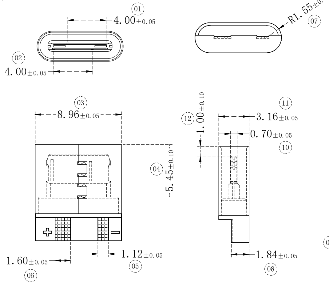
接点定义放大图(2P)
